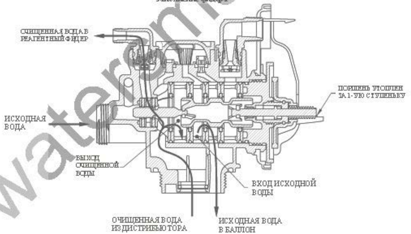
Заполнение фильтра
